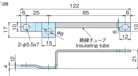
分岐銅帯接続例 (参考図)
