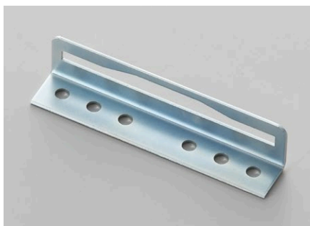
用途 盤用金具 サイズ 25W×20H×110L×1.6t 材質 SPCC
