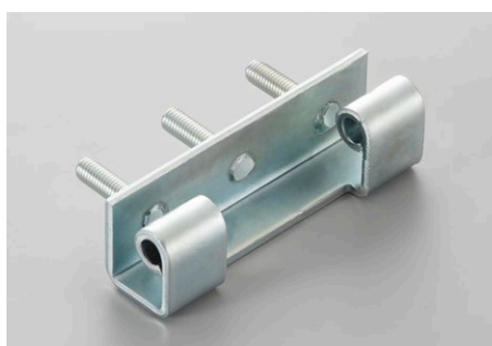
用途 大型盤用 サイズ 35W×135L×4.5t 材質 SPHC
